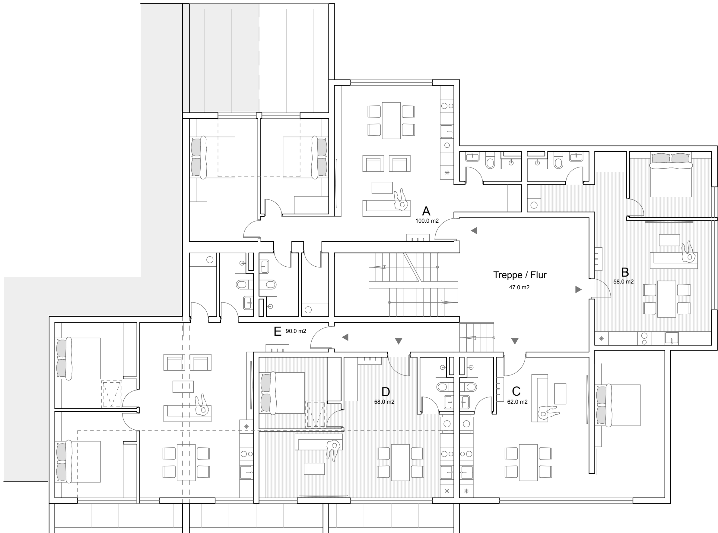
Grundriss 1 OG M 1:100 / 415.0 m²
